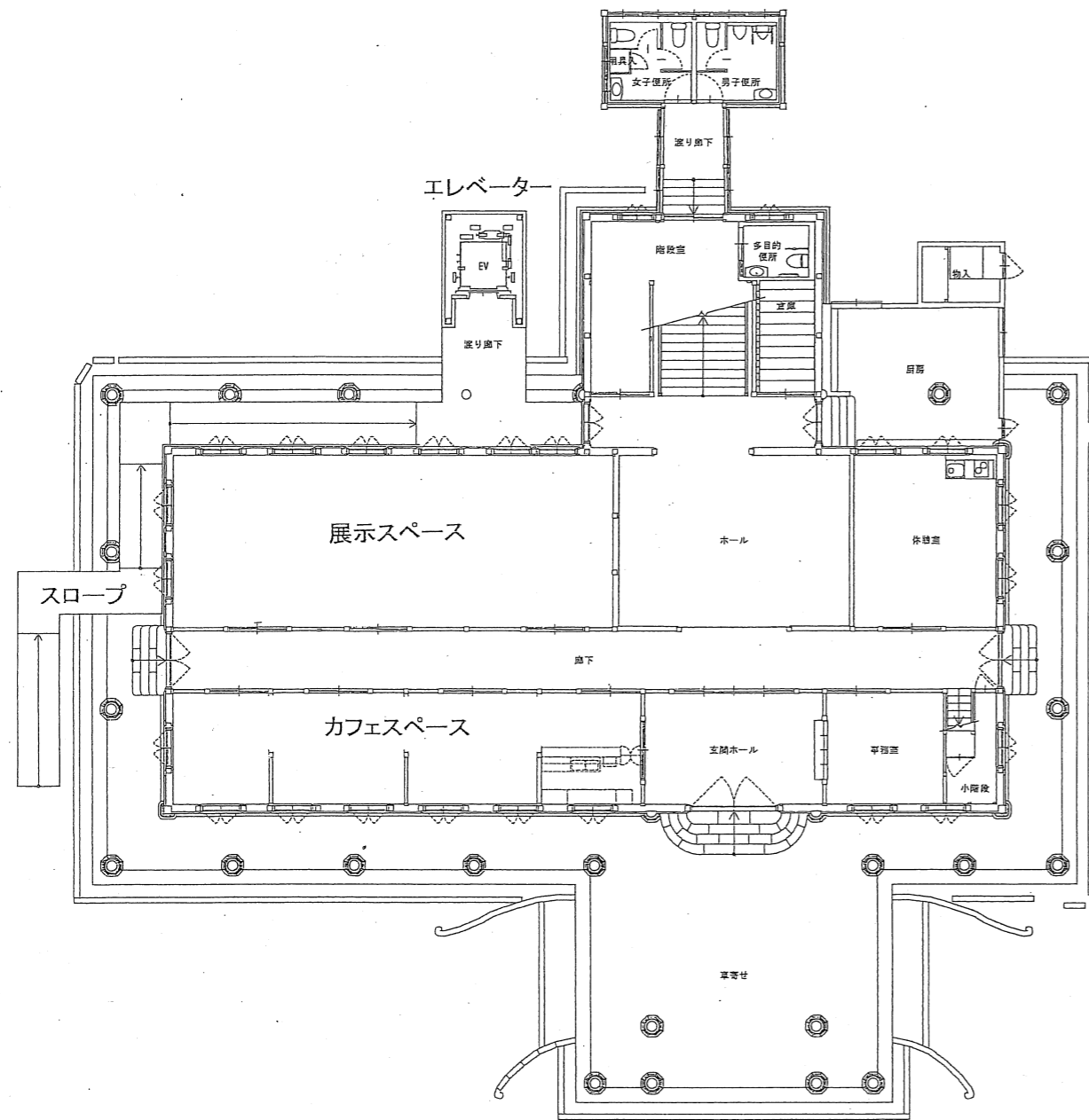
一階平面図
