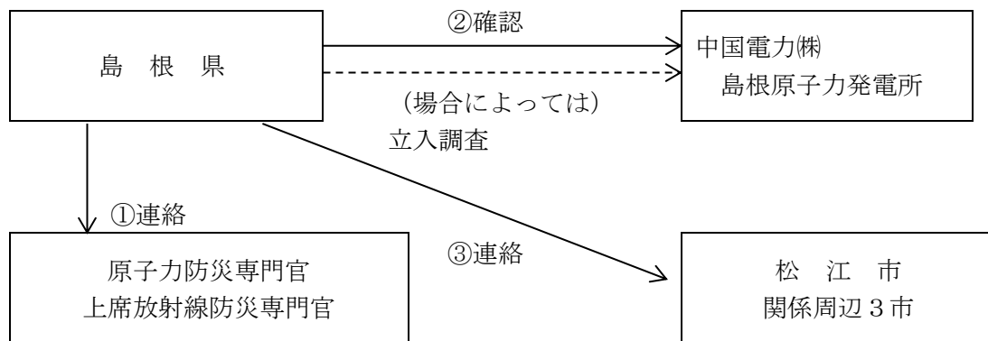
図 4-2-2 県モニタリングポスト（固定局）で施設敷地緊急事態（特定事象）発生通報を行うべき数値の検出を発見時の連絡系統図
